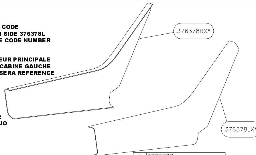
CABIN BOTTOM SIDE - 376 - FLANC DE CABINE INFÉRIEUR
