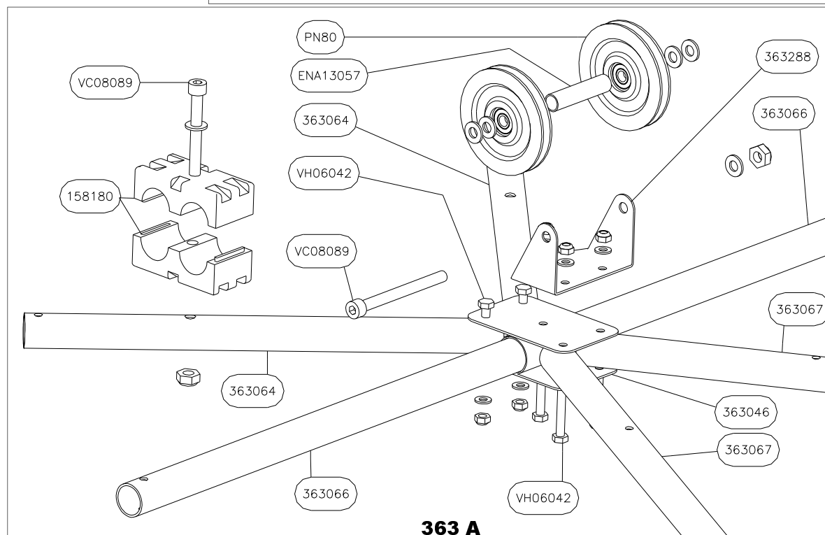
UNDER SEAT TUBES FRONT - 363 - TUBES SOUS SIEGES AVANT
