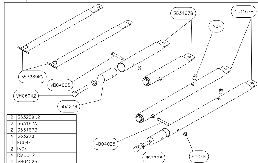
CABIN ENTRY DIAGONAL TUBES - 353 - TUBES RAIDISSEURS D'ENTREE CABINE Type 2
