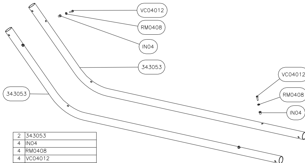
DOOR ENTRANCE TOP - 343 - TUBE ENTREE CABINE HAUT
